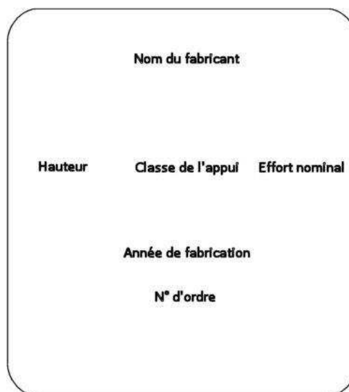
Figure 1 - Marquage sur poteau béton
