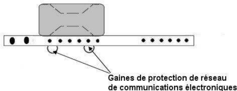
Figure 10 - Liaison aéro-souterraine sur poteau béton
