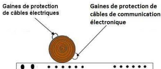
Figure 11 - Liaison aéro-souterraine sur poteau bois
